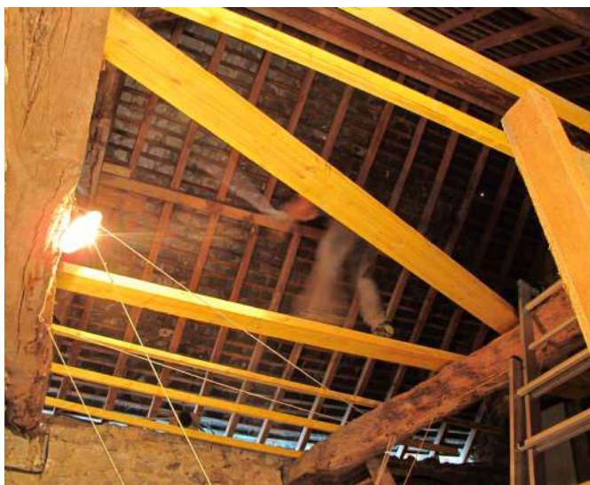
Pose de l'ossature
